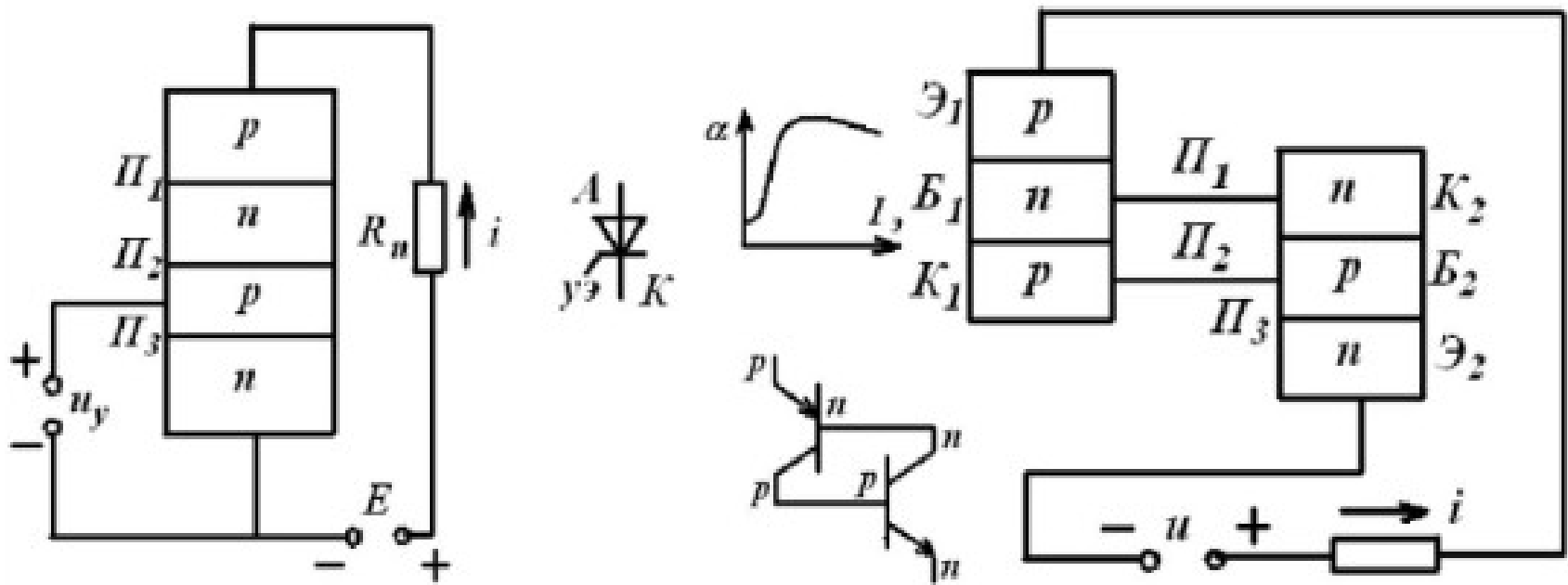
Рисунок 16. Структурная схема тиристоров
